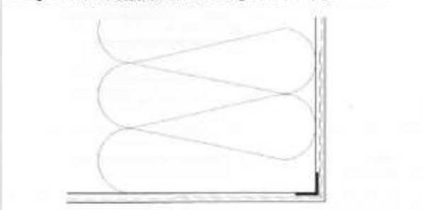
Dettaglio costruttivo: sezione orizzontale di angolo con parasigolo con rete
