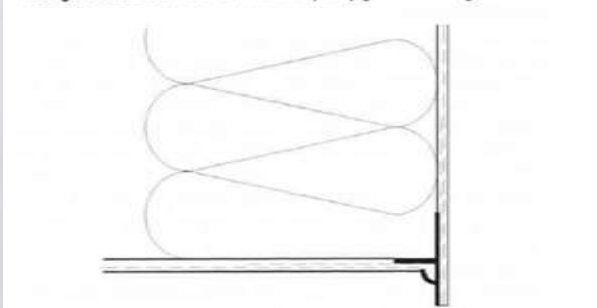
Dettaglio costruttivo: sezione verticale con parasigolo con rete e gocciolatoio
