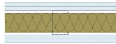
Parete SUPER 125/75 mw
