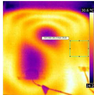
Ore 12:05 - Massetto tradizionale Temperatura media area = 29,1°C
