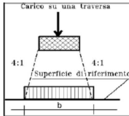
Fig. 5.2.4 - Distribuzione longitudinale dei carichi attraverso il ballast
