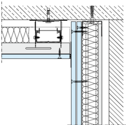
NODO CONTROSOFFITTO – CONTROPARETE
