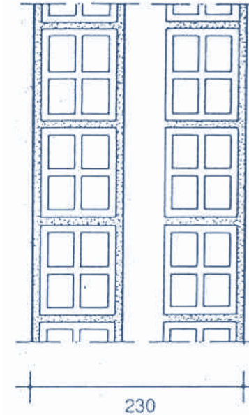
MURATURA DOPPIA
