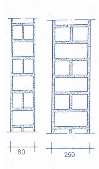
MURATURA SEMPLICE
