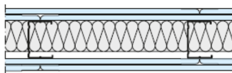
W112 Parete a singola orditura doppio rivestimento per lato
