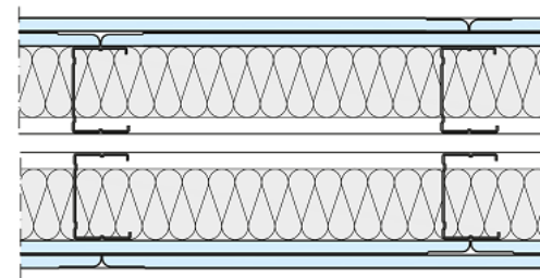
W115 Parete doppia orditura affiancata Doppio rivestimento per lato
