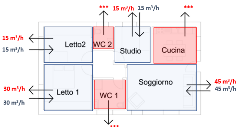
Schema per la ripartizione delle portate di progetto
